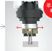
挿入時の 芯ズレ吸収
