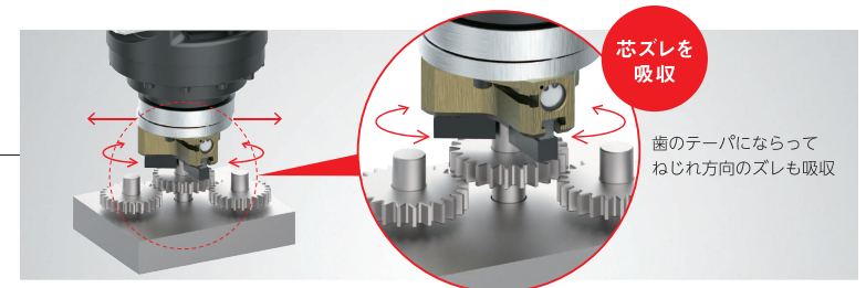
ワークとロボットアームの 中心にズレ
